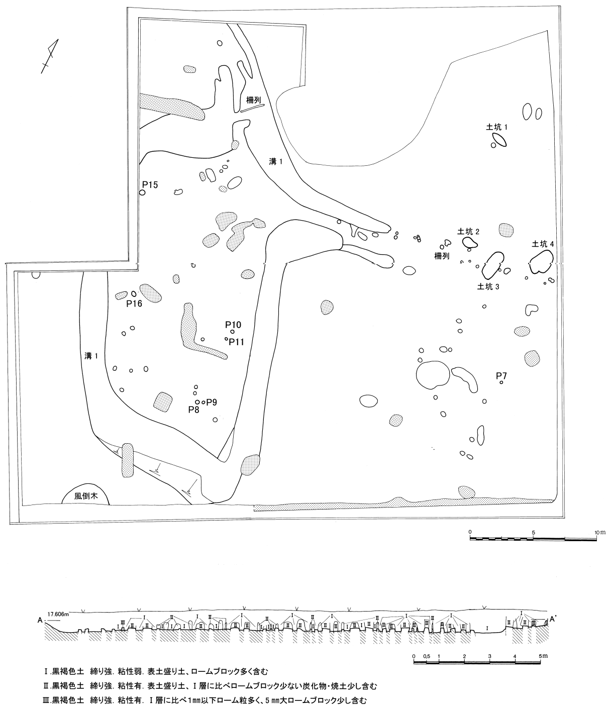
第47図 本村遺跡第117地点遺構配置図 (1/300)、土層 (1/150)
