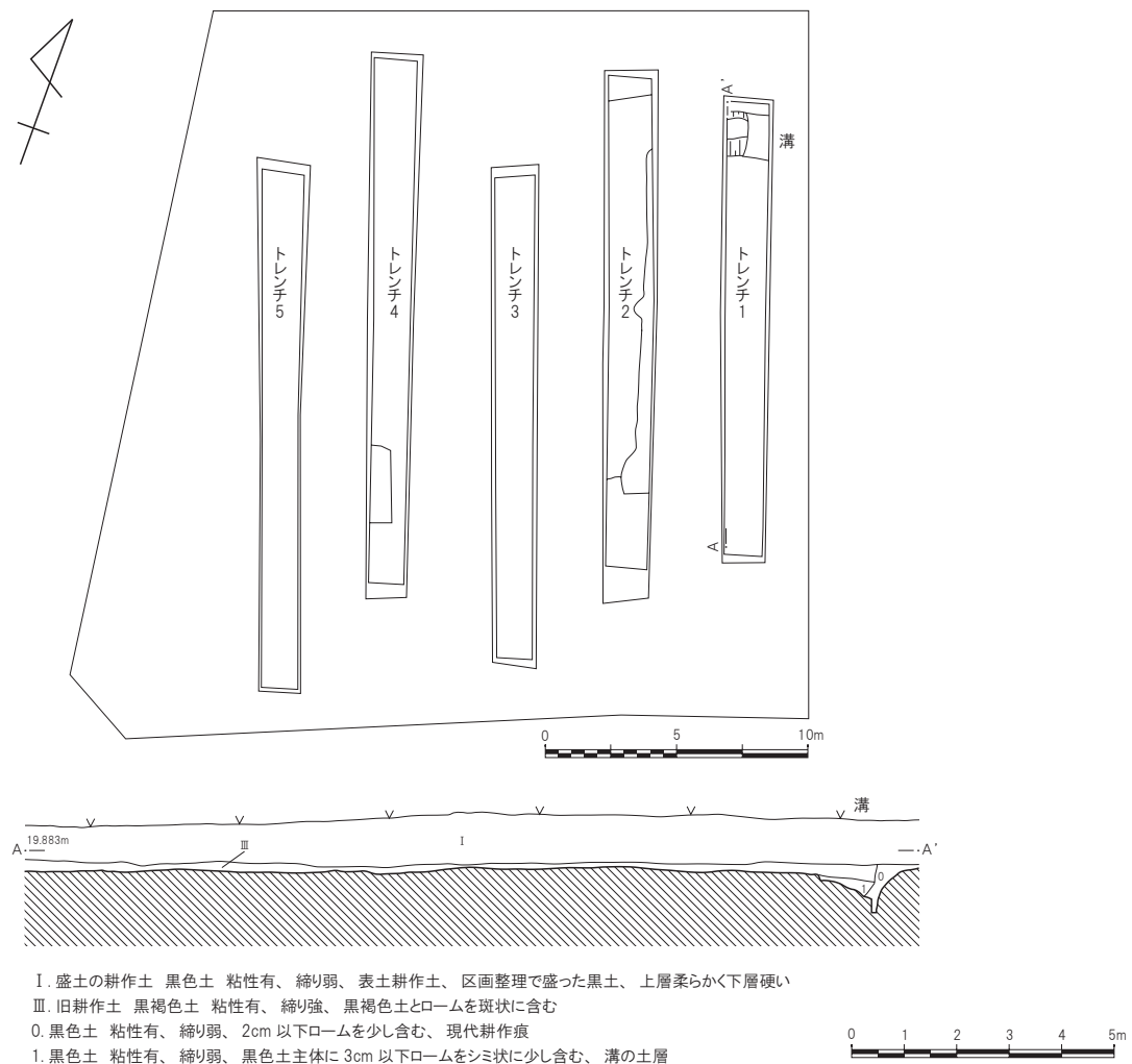
第 47 図 本村遺跡第 140 地点遺構配置図 (1/300)、土層 (1/150)
