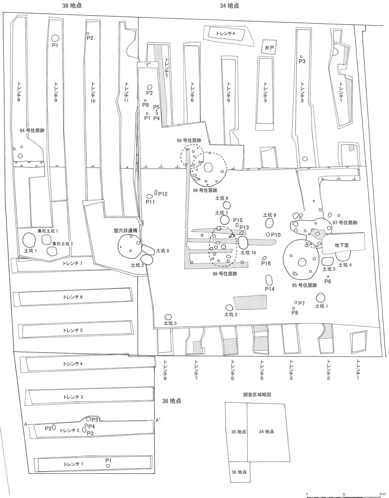
第75図 東台遺跡第34・36・38地点遺構配置図 (1/300)
