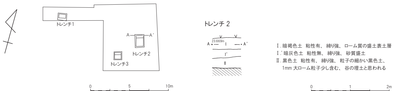
第 49 図 東台遺跡第 63 地点遺構配置図・第 64 地点調査区域図 (1/300)、第 63・64 地点土層 (1/60)
