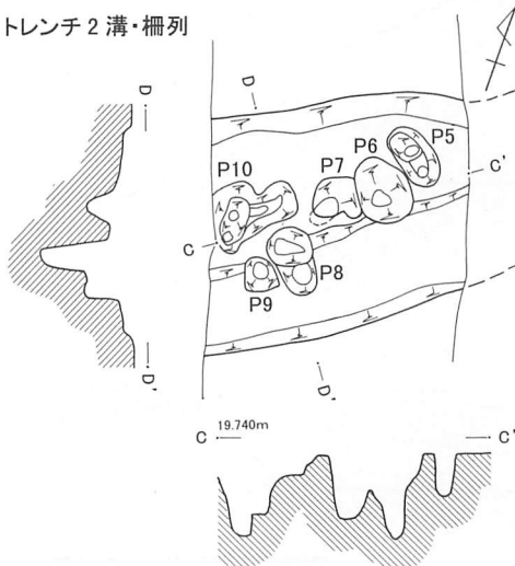
第28図 亀久保堀跡遺跡第26地点遺構配置図 (1/300) 土層・溝・柵列 (1/60)
