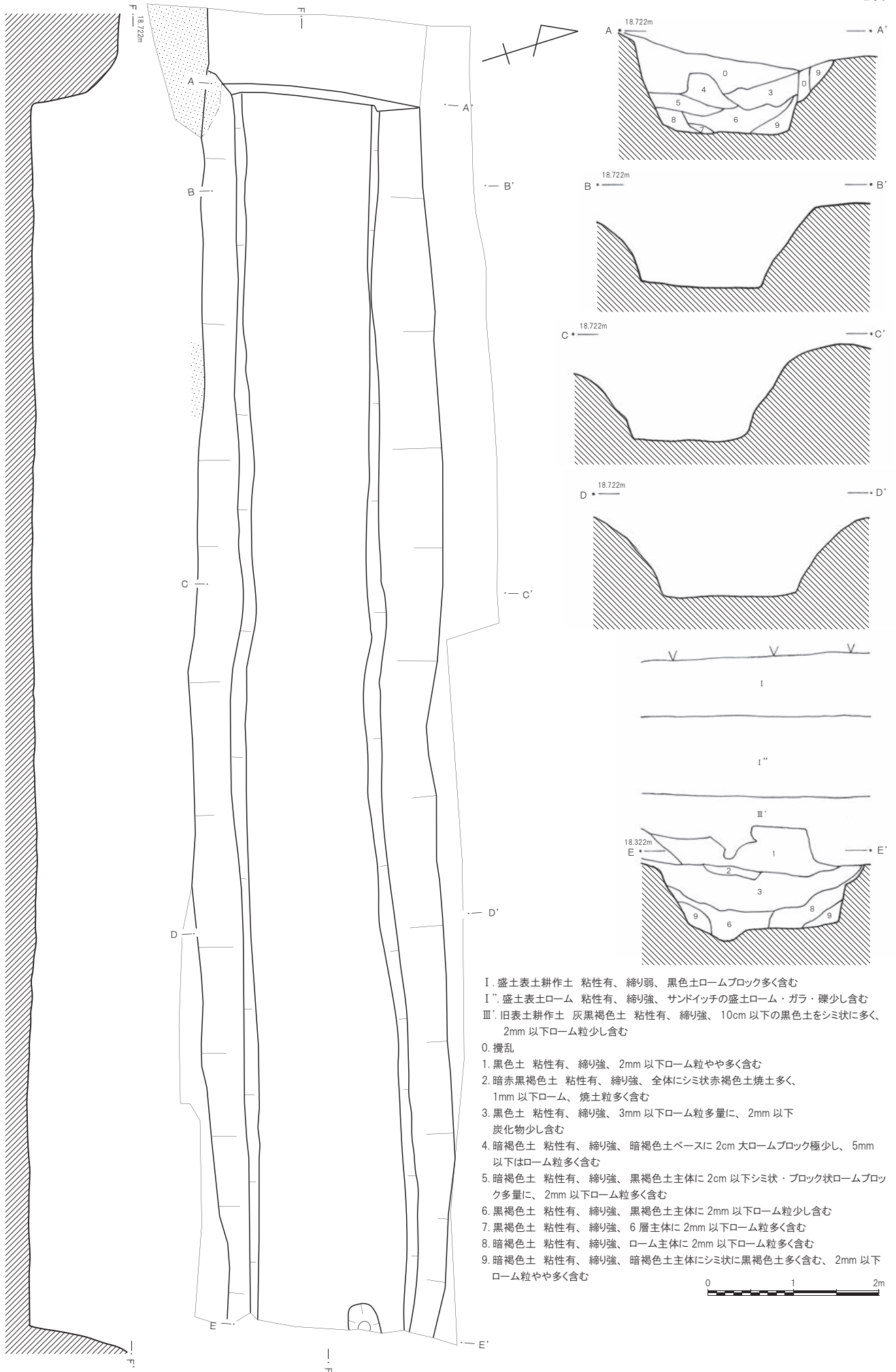
第70図 亀久保堀跡遺跡第34地点堀跡(1/60)
